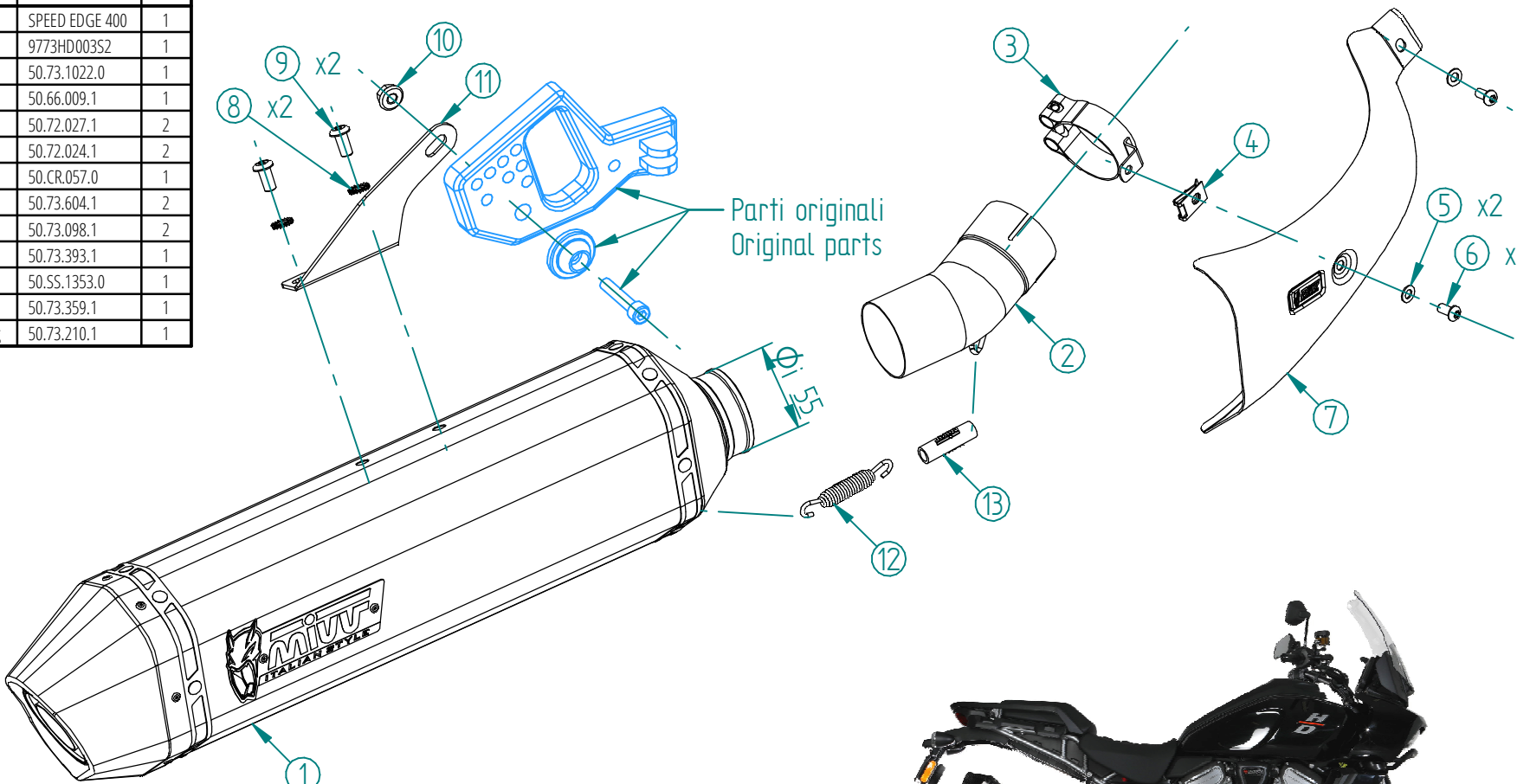
Collettore 2in1 / 2in1 header pipe
