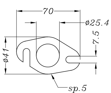
Vista da "A" Flangia "96A"
